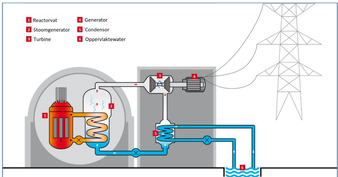
Figuur 5: Schematische weergave van een kerncentrale
