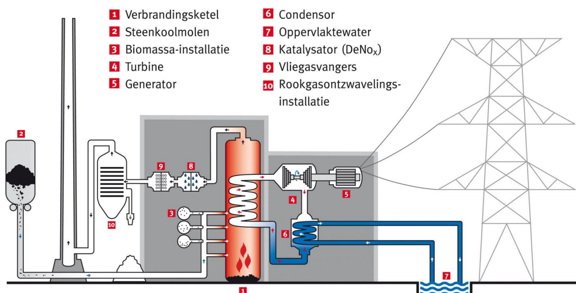
Figuur 11: Schematische weergave van een kolencentrale
