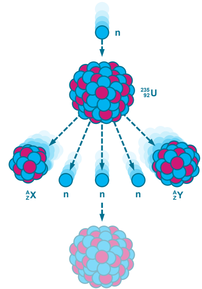
Figuur 4: Voorbeeld van een kernsplijting van een uraniumkern
