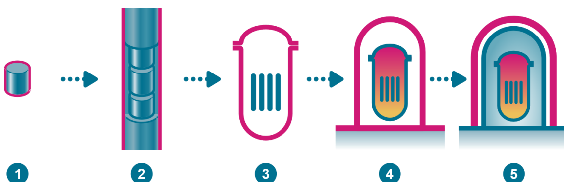
Figuur 16: De veiligheidslagen van een kerncentrale
