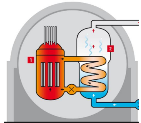
Figuur 6: De reactorkern en stoomgenerator in een kerncentrale
