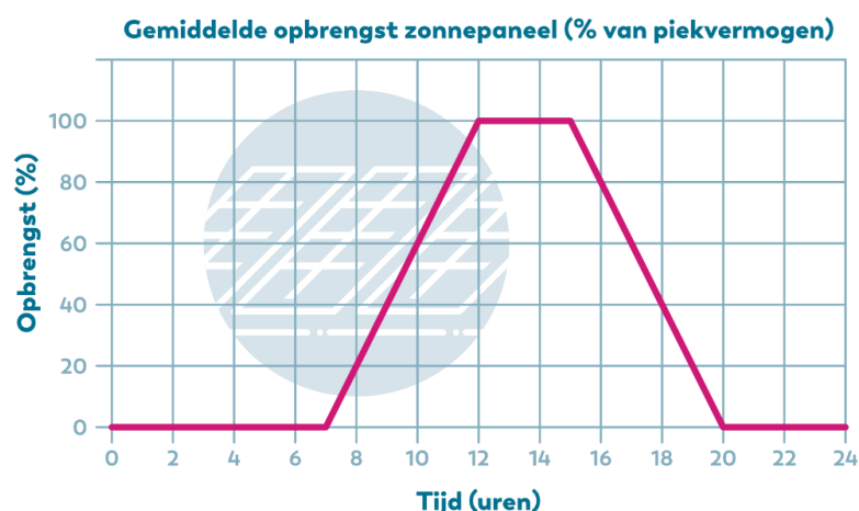
Figuur 9: Voorbeeldopbrengst van een zonnepaneel op een dag (% van piekvermogen)
