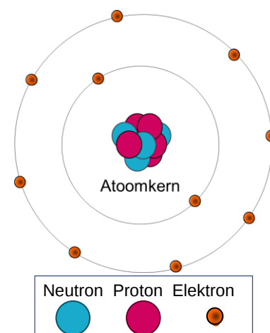
Figuur 2: Atoomkern met elektronen
