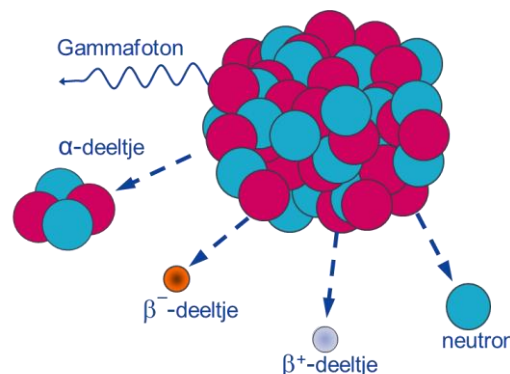
Figuur 3: Verschillende vormen van radioactief verval.
